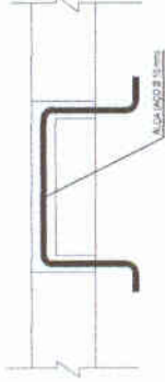
DETALHE DA ALCA ESC:1
