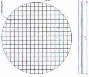
FOSSA SÉPTICA FUNDO EM CONCRETO ARMADO ESC:1/2
